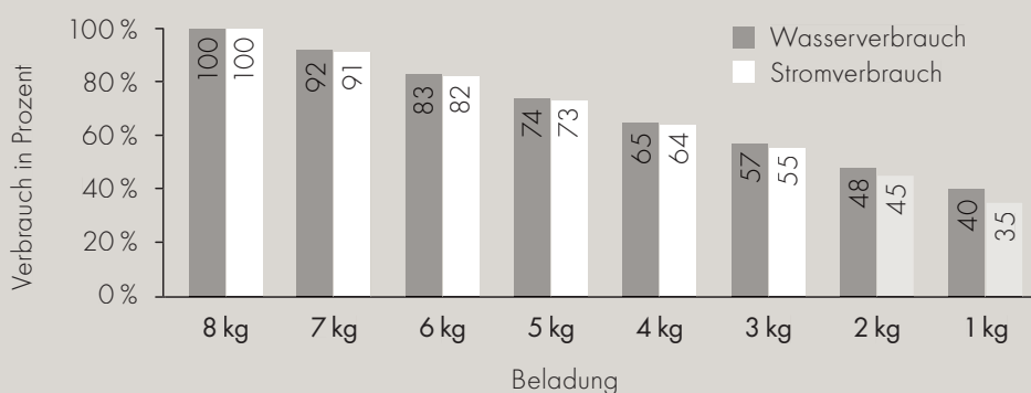
Einsparung durch Teilbeladungs-Sparautomatik
