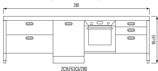
Elemento con pannello per lavastoviglie e forno da 60 cm Element mit Abdeckplatte für Geschirrspüler und Backofen 60 cm
