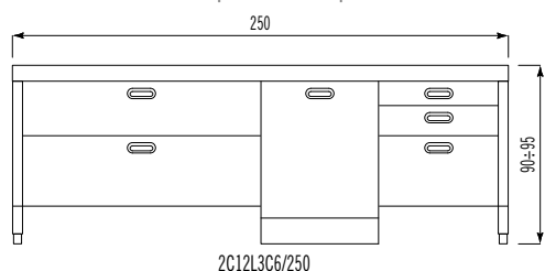
Elemento con pannello per lavastoviglie Element mit Geschirrspüler-Abdeckplatte
