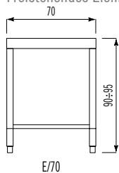
Elemento libero Freistehendes Element
