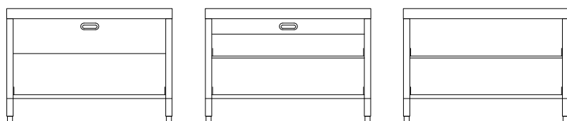
Elemento aperto con ripiani scorrevoli 120 cm Offenes Element mit Gleitablagen 120 cm
