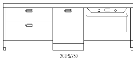
Elemento con pannello per lavastoviglie e forno da 90 cm Element mit Abdeckplatte für Geschirrspüler und Backofen 90 cm
