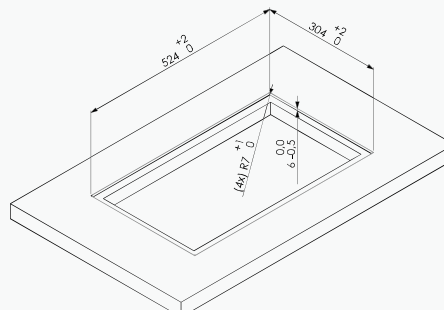
Flächenbündiger Ausschnitt
