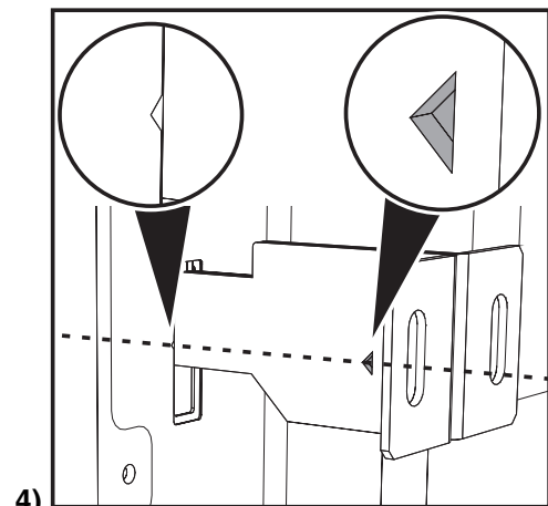
4) Bevor die Bügel an der Wand vollständig festgeschraubt werden, prüfen, ob sich die Markierung an den Bügeln auf der gleichen Höhe der Markierung hinten am Gerät befindet. Bei Positionierung des Gerätes darauf achten, dass die Bügel richtig eingehakt werden.
