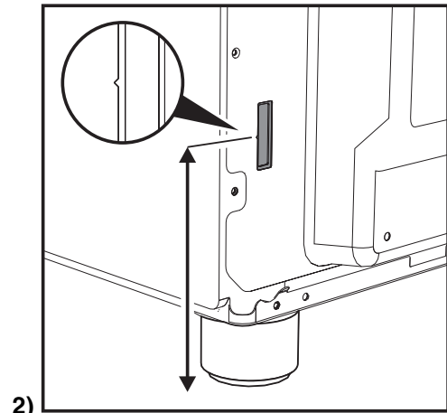
2) Den Abstand zwischen der Anzeige des Spaltes und dem Boden messen.
