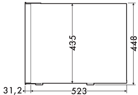
(Seitenansicht)
